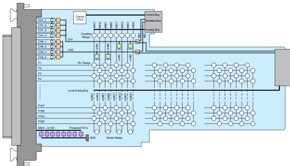
Abbildung 1: Blockschaltbild
